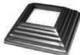
ОС50 Основание стойки Размеры: 100*30, □50*50 (1мм) Цена : 50руб
